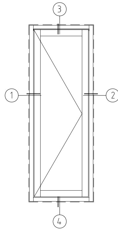
HINGED DOOR
